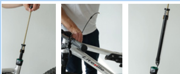
Illustration 165 : Retirer la cartouche
