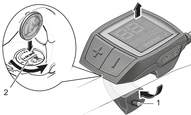
Illustration 131 : Ordinateur de bord avec vis de fixation (1) et couvercle du logement des piles (2)
