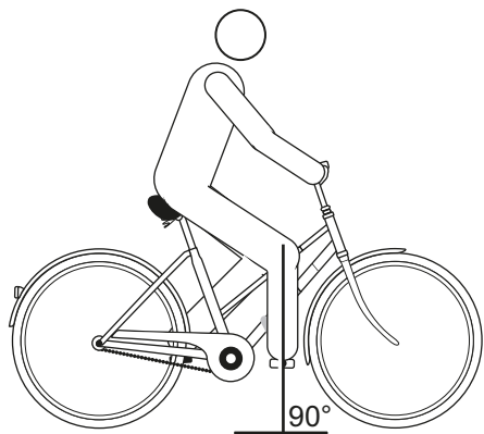
Illustration 92 : Verticale de la rotule
