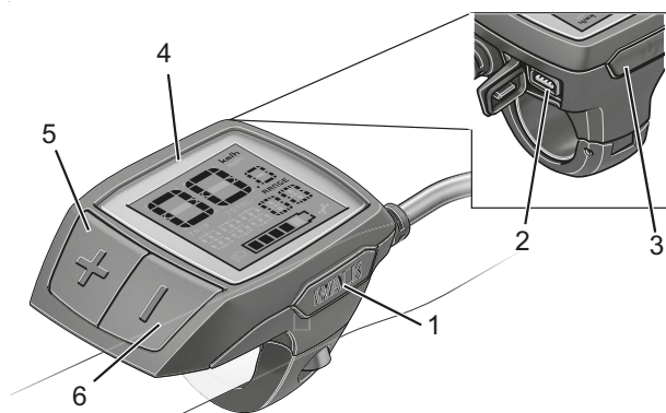
Illustration 40 : Structure de l'ordinateur de bord BOSCH Purion
