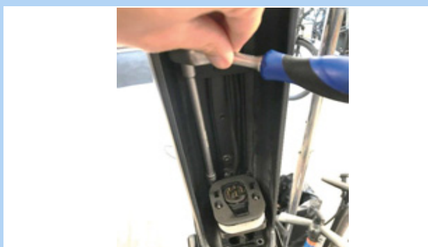
Illustration 55 : Retirer les vis à six pans creux
