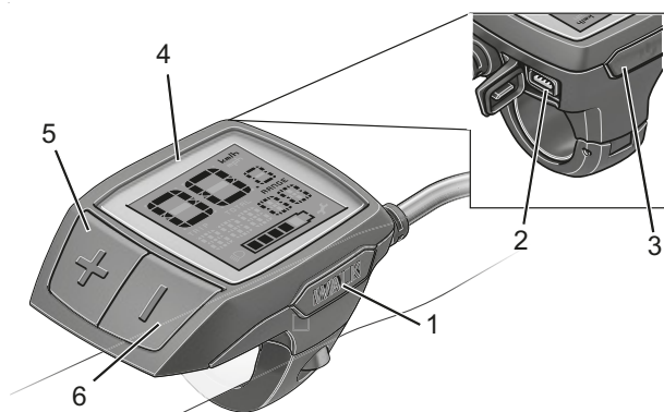
Illustration 130 : Structure de l'ordinateur de bord BOSCH Purion
