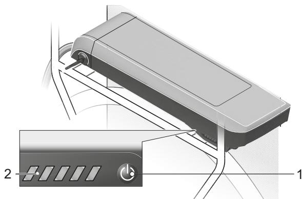
Illustration 48 : Position de l'indicateur de charge de la batterie pour porte-bagages
