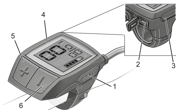
Illustration 117 : Structure de l'ordinateur de bord BOSCH Purion
