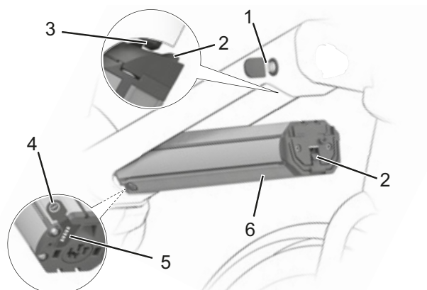
Illustration 37 : Détail d'une batterie intégrée
