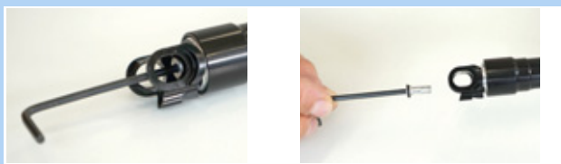
Illustration 181 : Retirer le capuchon de valve
