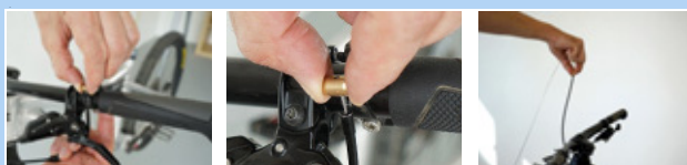
Illustration 173 : Détacher la télécommande
