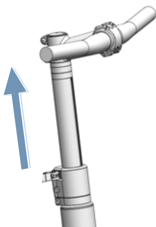
Illustration 115 : Exemple d'un All Up tiré dans la position la plus haute
