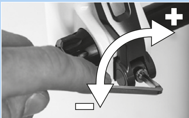
Illustration 52 : Régler la force de serrage de l'attache rapide
