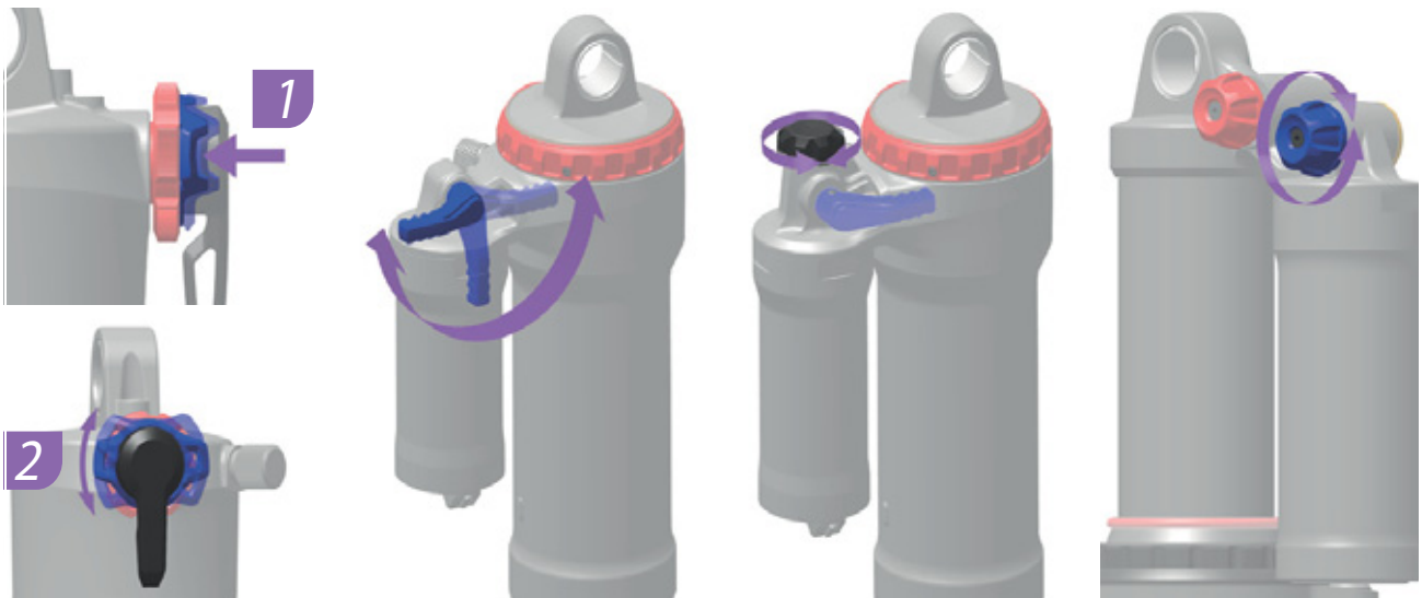
Illustration 225 : La position et la forme du dispositif de réglage de la compression (bleu) dépendent du modèle
