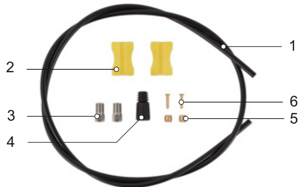
Illustration 20 : Composants de la ligne de frein
