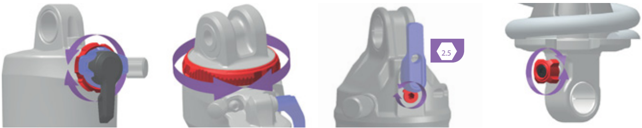
Illustration 221 : La position et la forme du dispositif de réglage de la détente (rouge) dépendent du modèle
