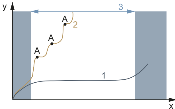
Illustration 117 : Diagramme d'usure, durée de service (x) par rapport à l'enlèvement de matière (y)
