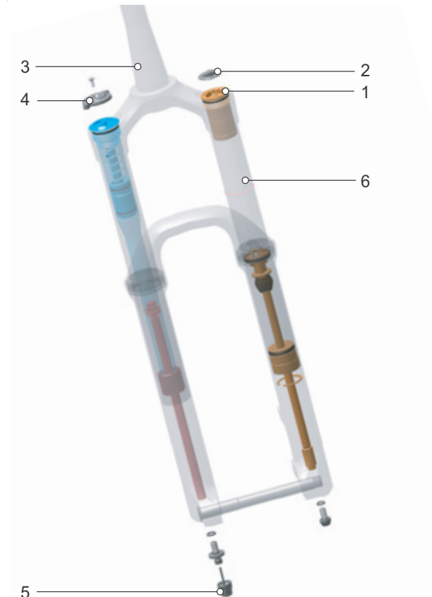
Illustration 13 : Structure interne de la fourche suspendue pneumatique
