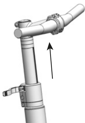
Illustration 72 : Tirer le levier de blocage vers le haut, exemple d'un All Up
