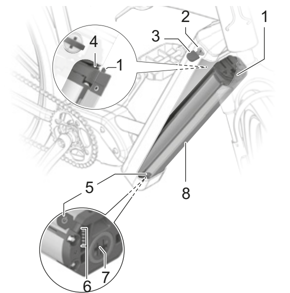
Illustration 29 : Détail de la batterie PowerTube 750
