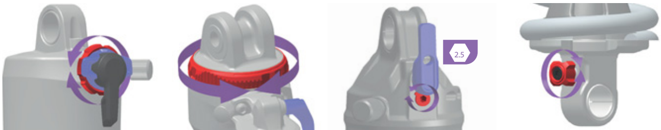
Illustration 223 : La position et la forme du dispositif de réglage de la détente (rouge) dépendent du modèle
