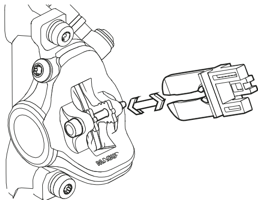
Illustration 37 : Insérer la cale de transport
